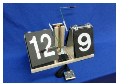
中国地域創造研究センター会長賞 「遠隔らくらく得点板」 広島大学附属中学校 第2学年 北野 愛翔
